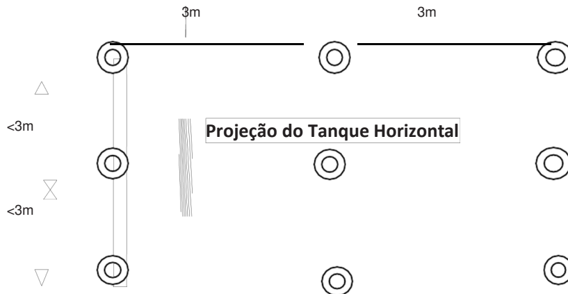
Figura 1 – Projeção do tanque aéreo horizontal com indicação dos pontos de medição de gases.
